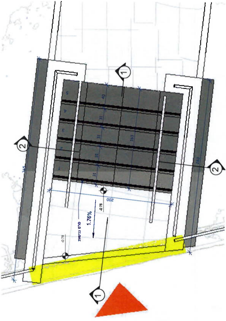
מדרגות(מזרחיות) עליה לפרגולה 1 : 25
